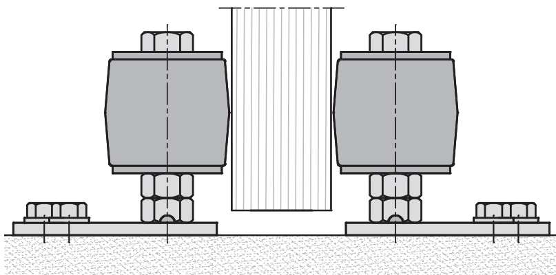
⑥ Bodenführungsrolle mit Platte
