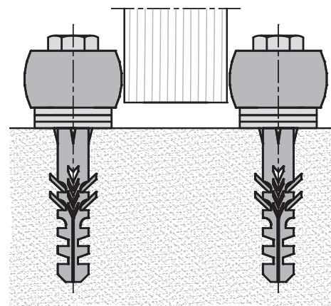
⑦ Außenführungsrolle mit Dübel
