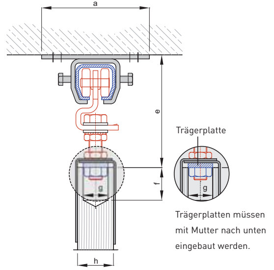
Deckenbefestigung
