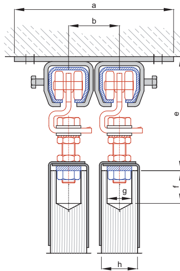
Doppeldeckenbefestigung
