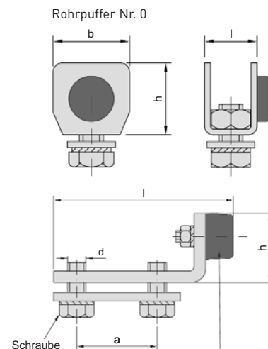
Rohrpuffer Nr. 1, Rohrpuffer Nr. 2
