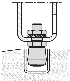
⑤ Bodenführungsrolle zum Schrauben
